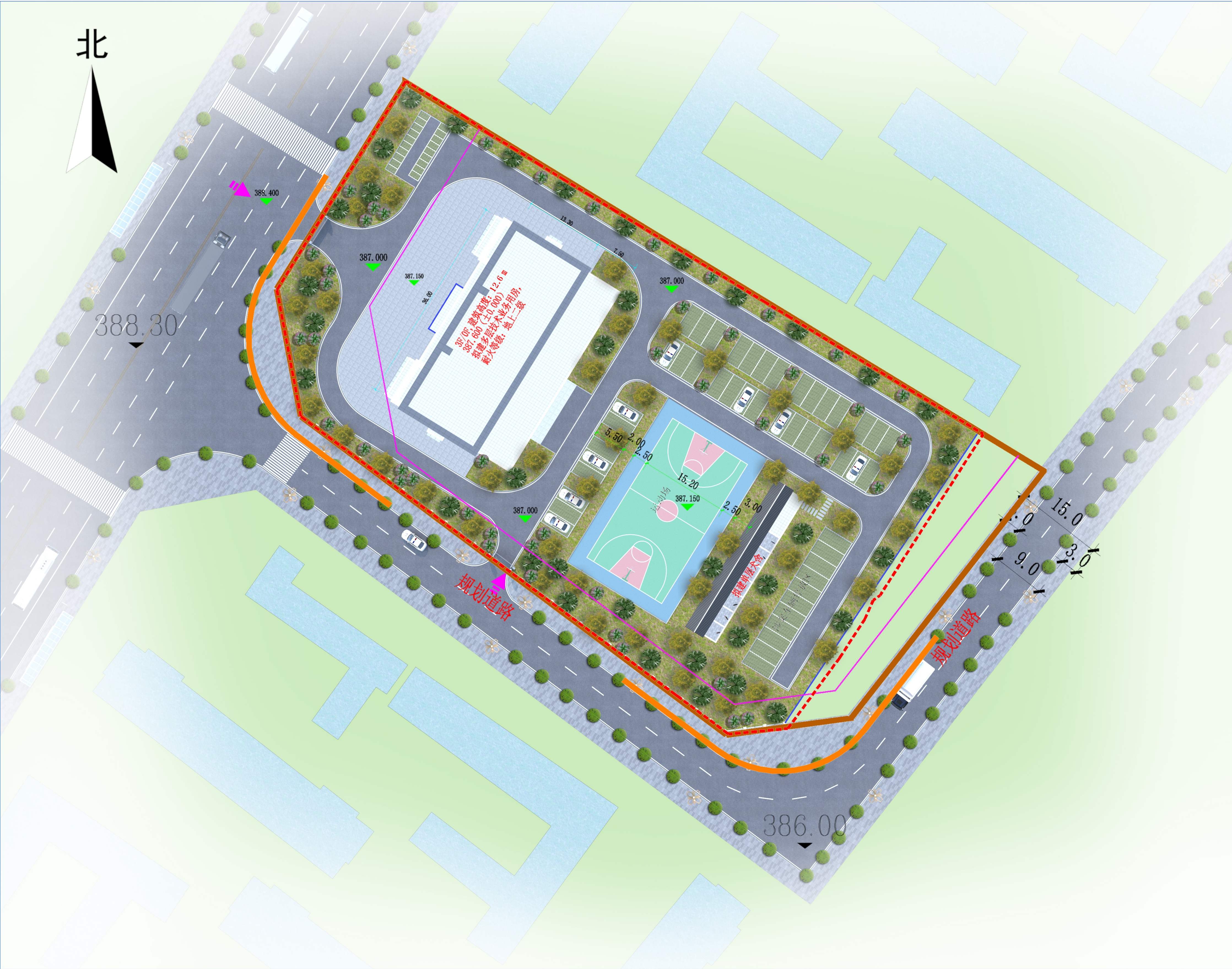
总平面图
