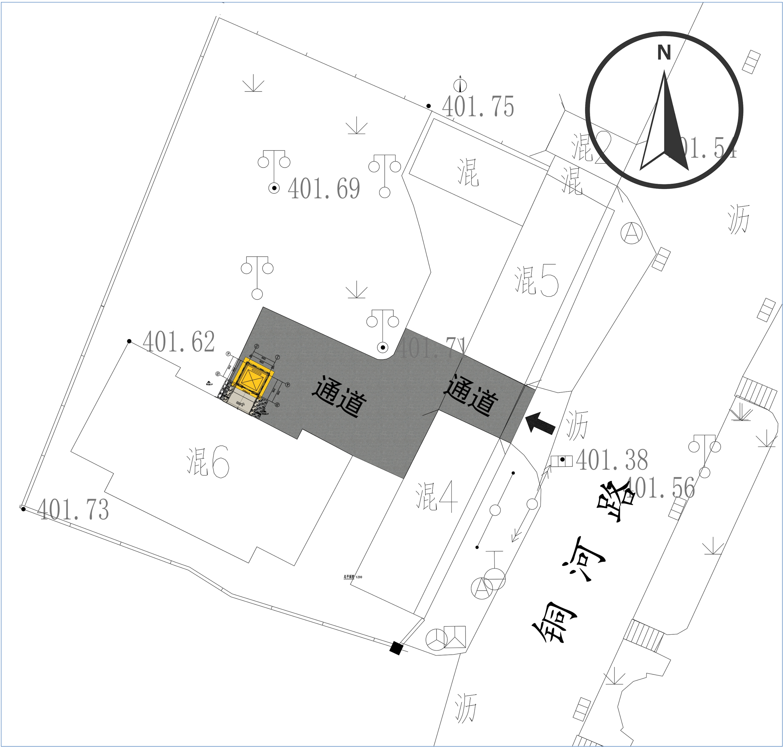
总平面图
