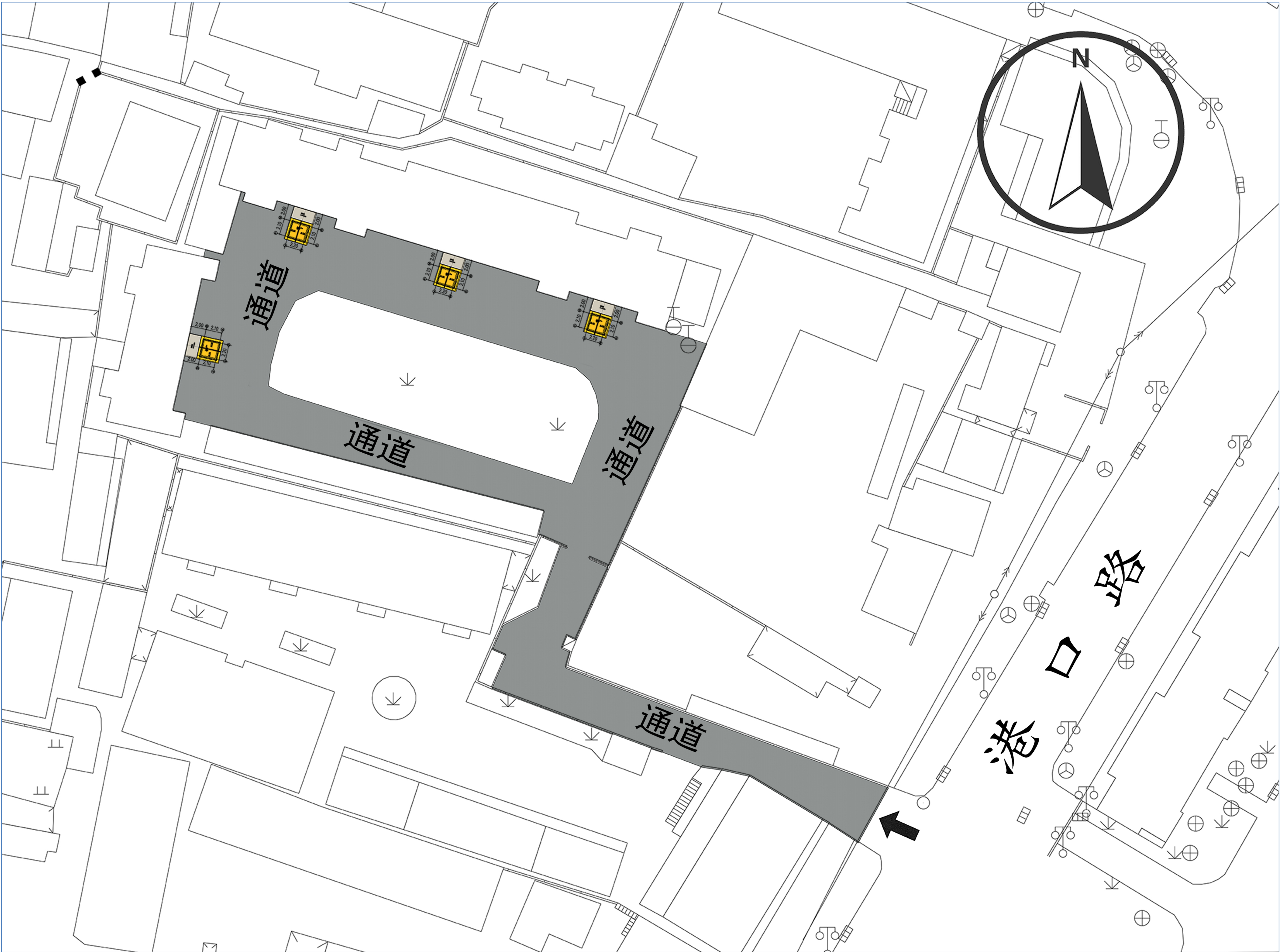
总平面图
