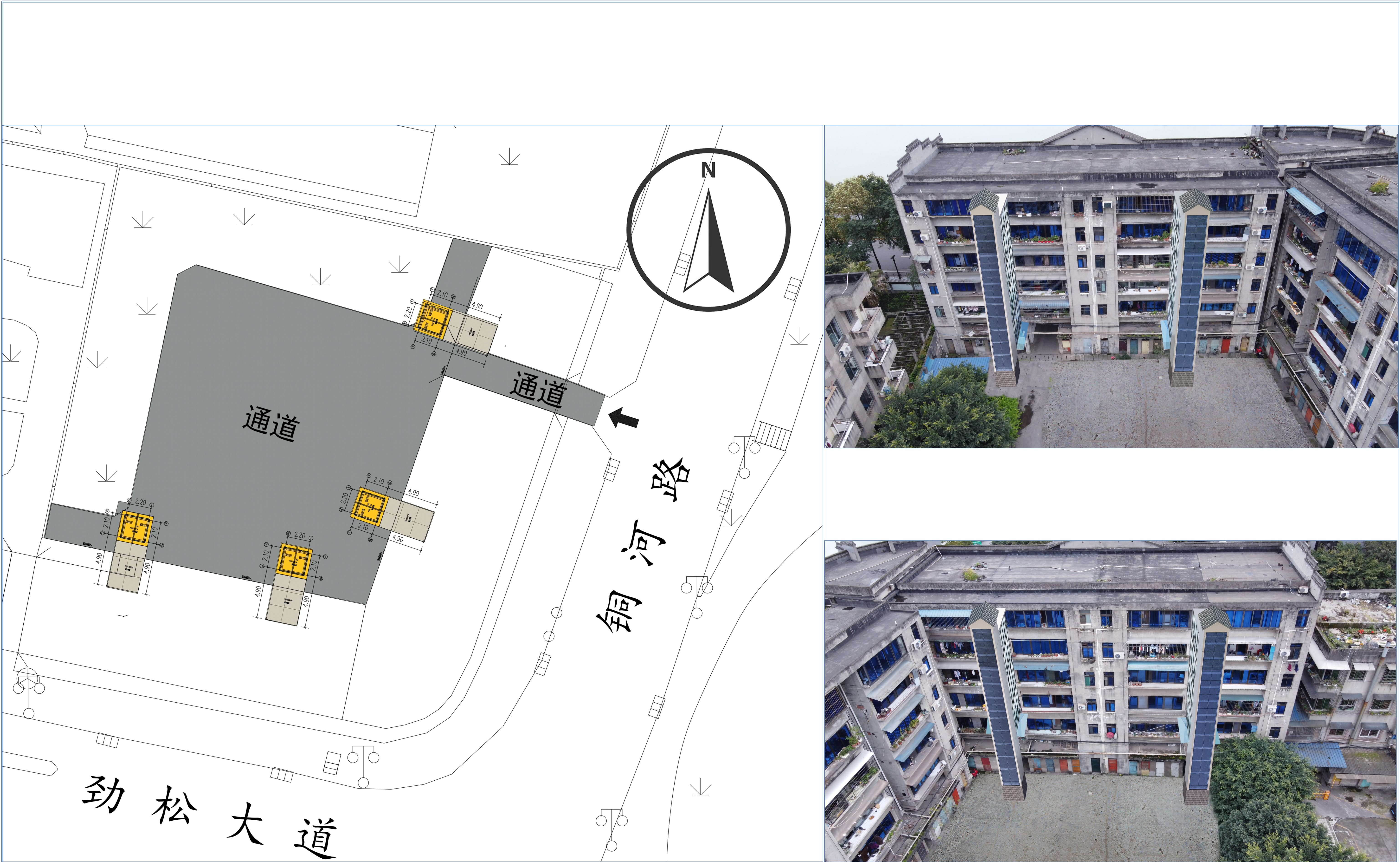
总平面图
