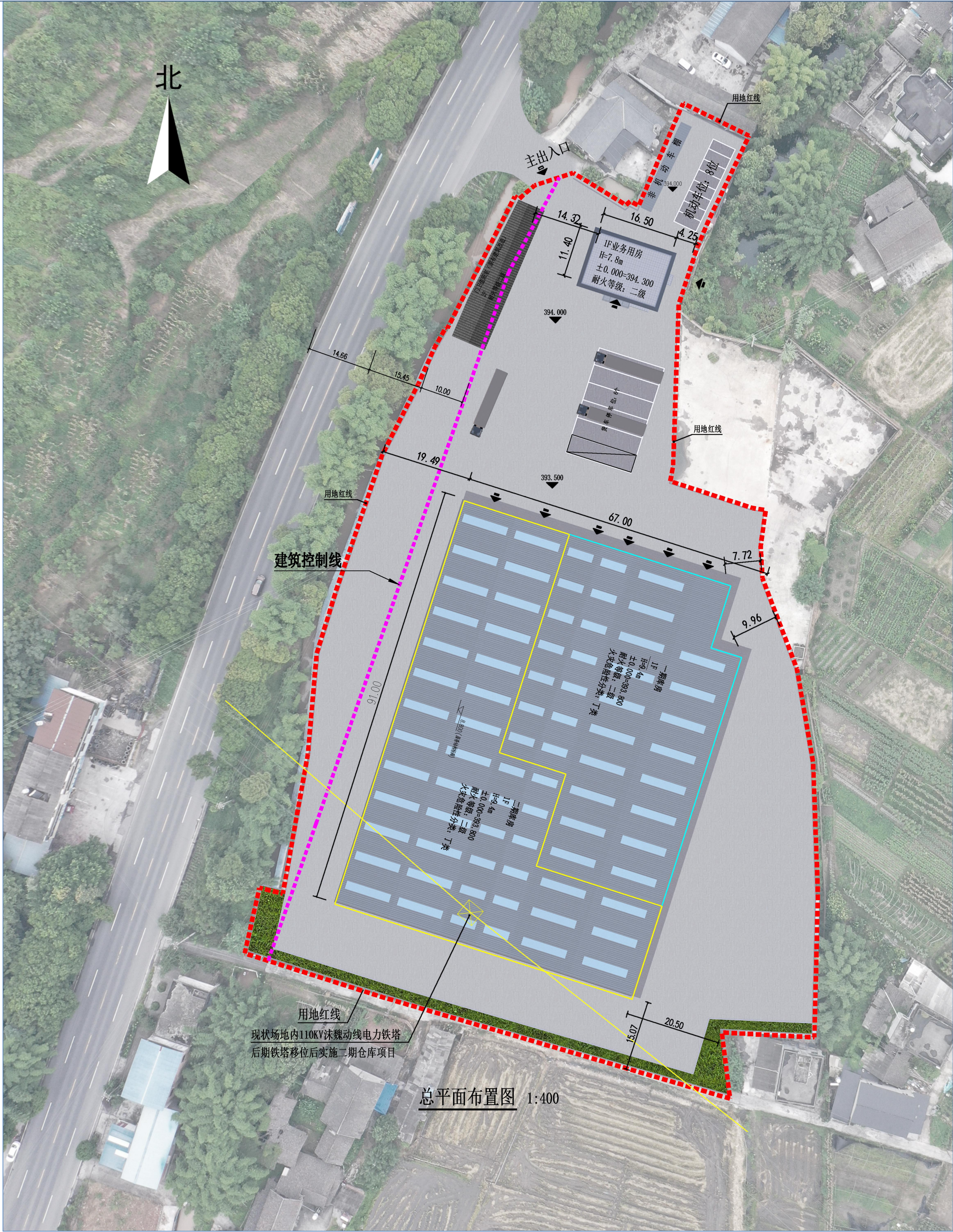
总平面图
