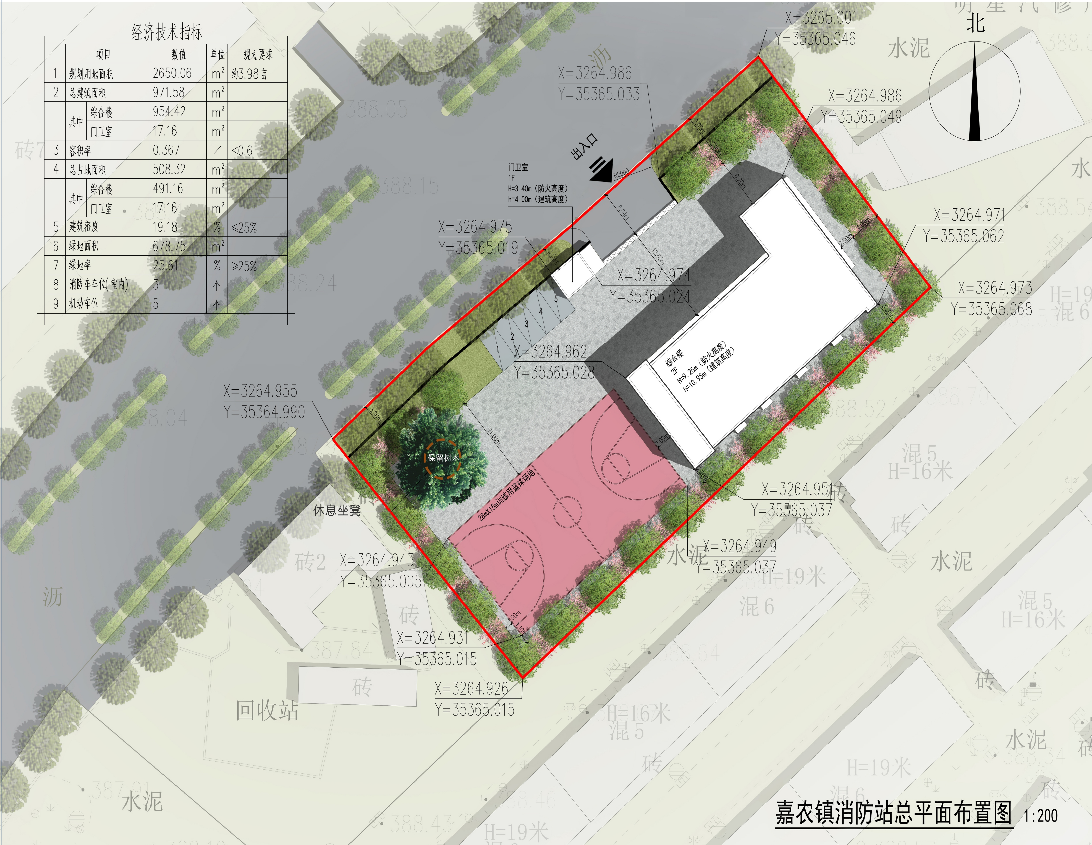
总平面图
