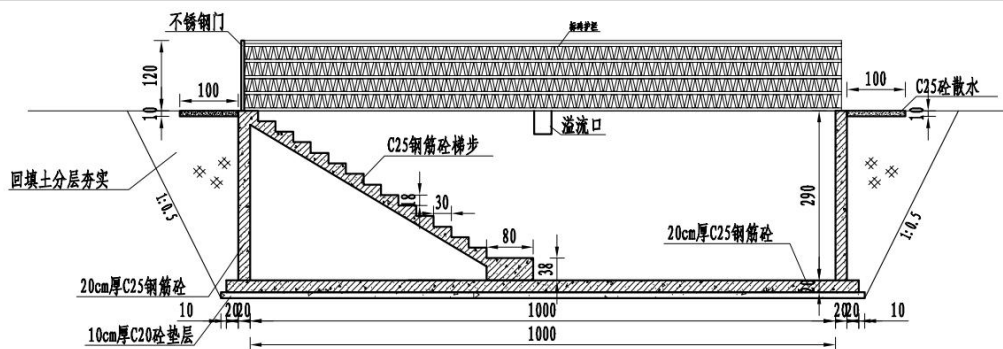
图 2-26 200m³蓄水池 B-B 剖视图
