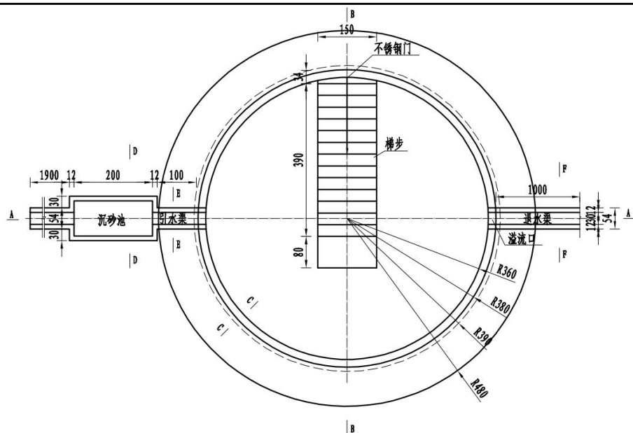
图 2-21 100m³蓄水池平面图
