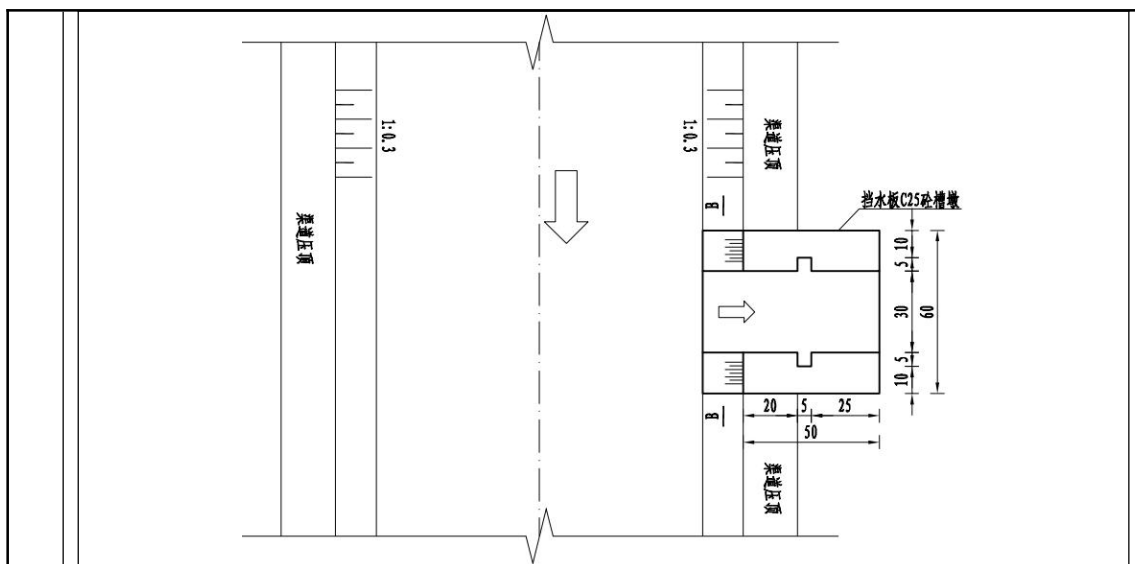
图 2-11 分水口平面图
