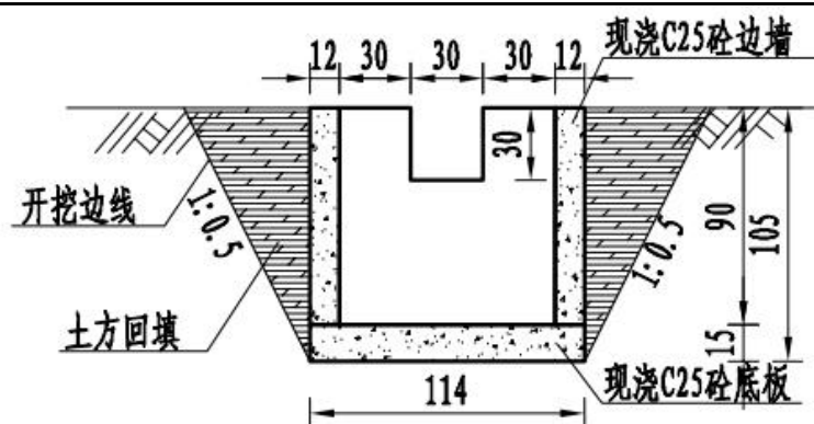
图 2-27 沉砂池剖面图
