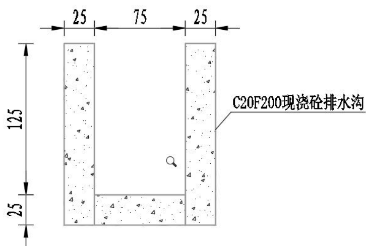
图 2-18 引水沟设计图
