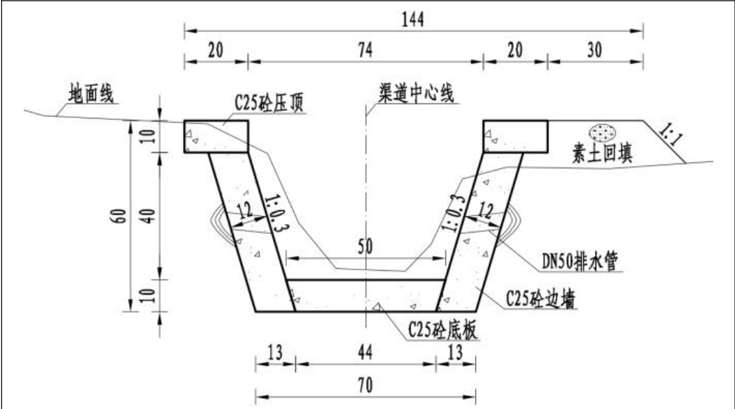
图 2-5 0.5m×0.5m 渠道典型横断面图
