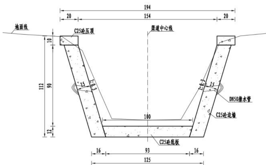
图 2-9 1.0m×1.0m 渠道典型横断面图
