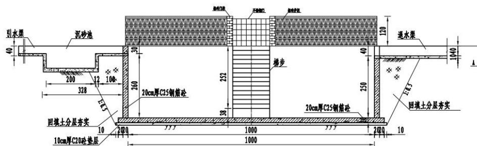
图 2-25 200m³蓄水池 A-A 剖视图
