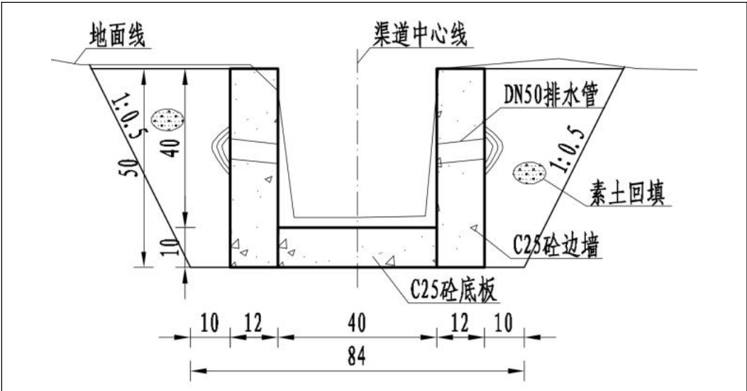
图 2-4 0.4m×0.4m 渠道典型横断面图
