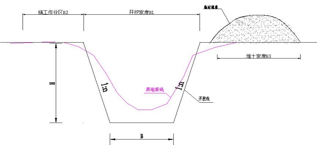
图 2-1 渠系工程及管道工程施工作业示意图
