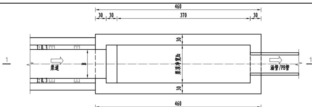
图 2-13 沉砂池平面图
