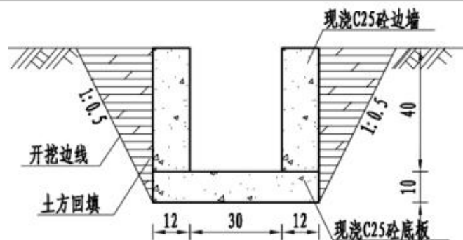
图 2-29 退水渠剖面图
