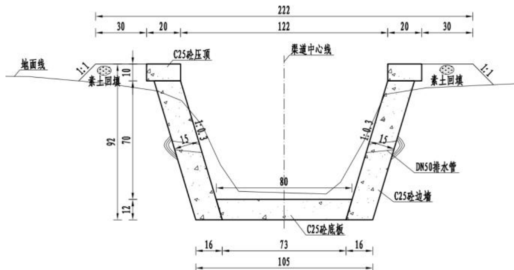
图 2-8 0.8m×0.8m 渠道典型横断面图
