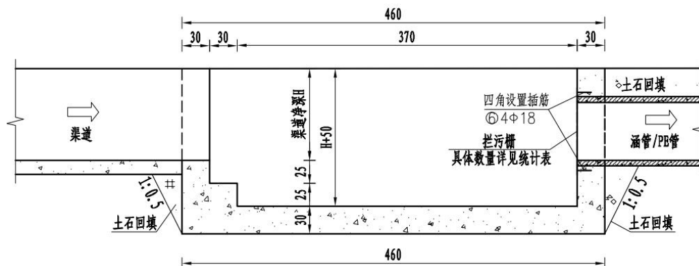
图 2-14 沉砂池 1-1 剖面图
