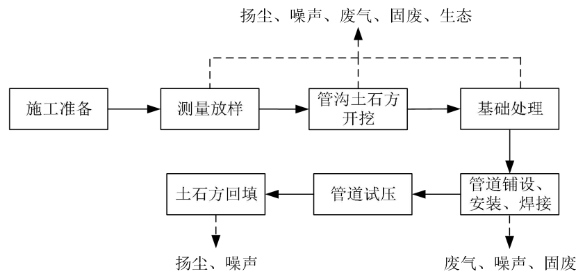
图 2-3 管道施工工艺流程及产污图
