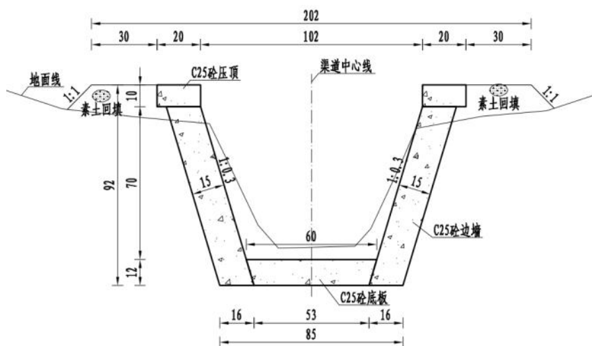
图 2-7 0.6m×0.8m 渠道典型横断面图
