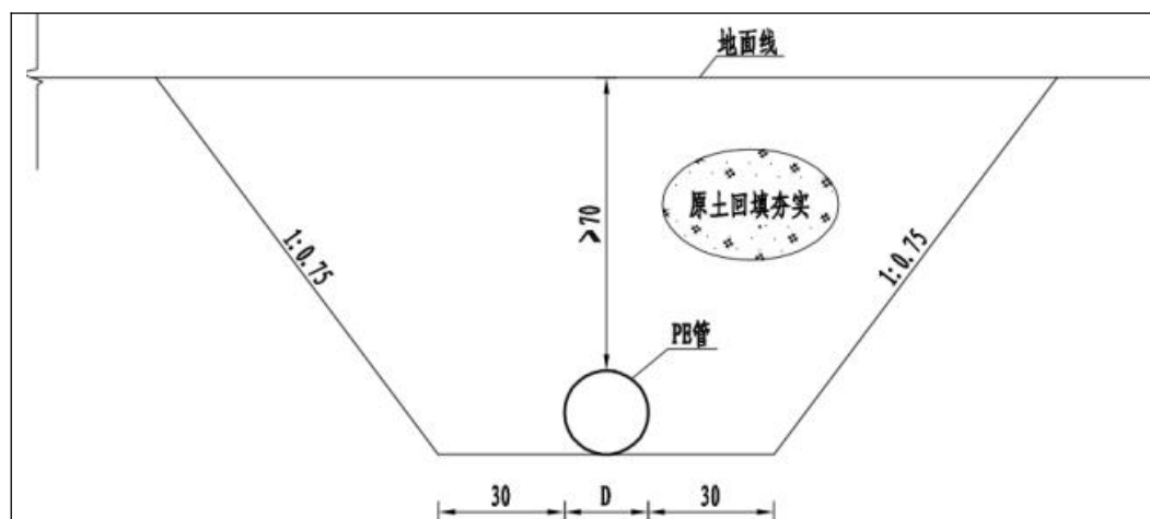
图 2-15 PE 管典型断面图
