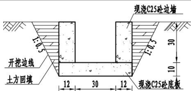
图 2-28 引水渠剖面图
