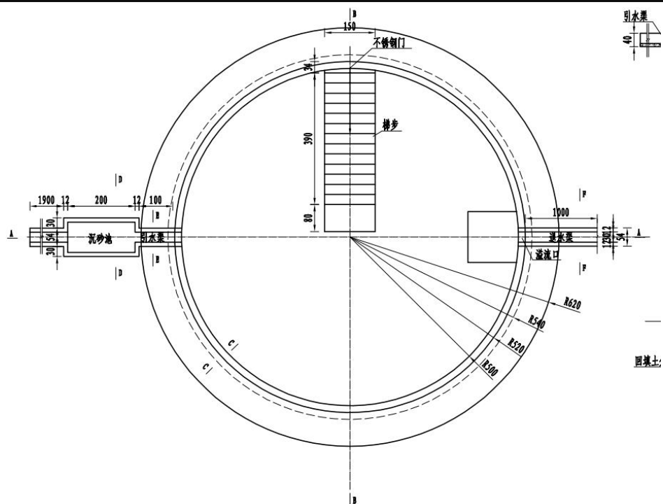
图 2-24 200m³蓄水池平面图
