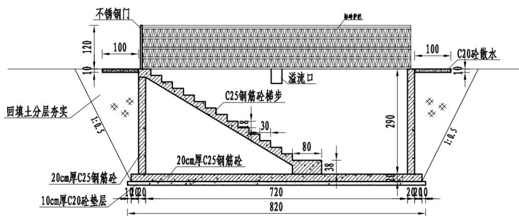
图 2-23 100m³蓄水池 B-B 剖视图
