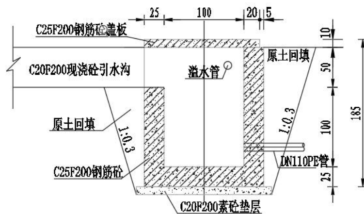
图 2-19 取水池剖面图
