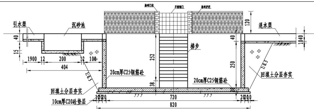
图 2-22 100m³蓄水池 A-A 剖视图
