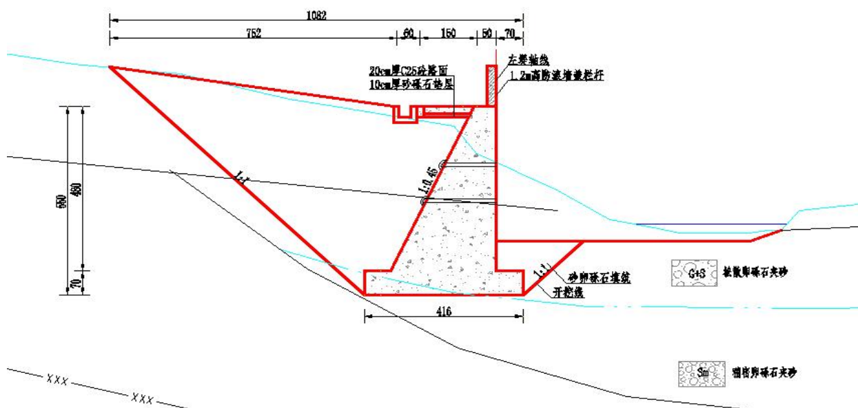
图 2-5C25 砼重式挡墙护岸
